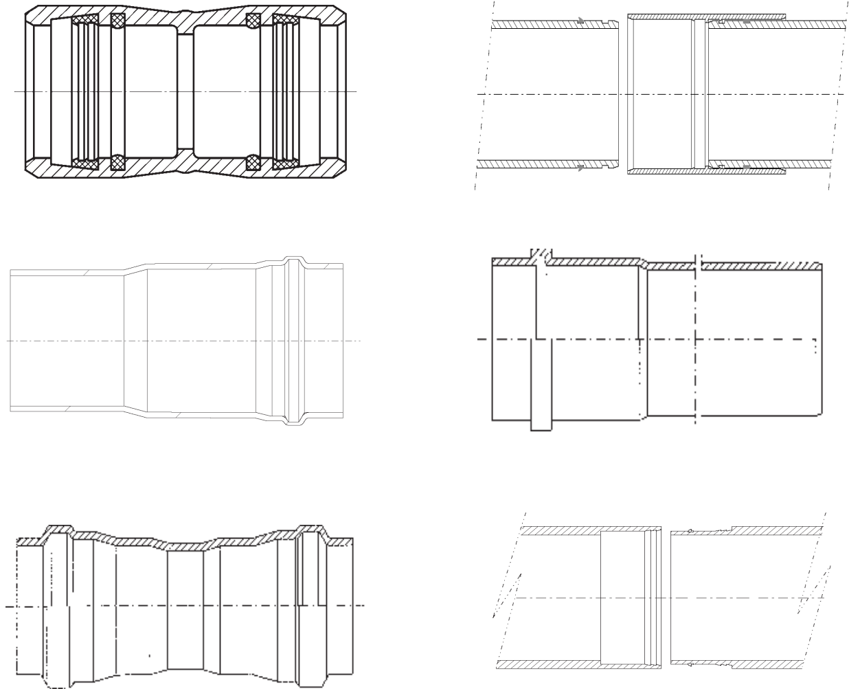
Elastomergedichtete Verbindungen
